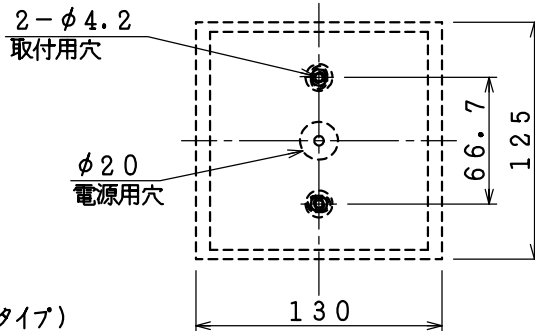
取付寸法(矢視⑧)
