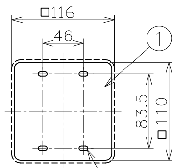
取付寸法（矢視 (a)） 2-5×10取付用長穴
