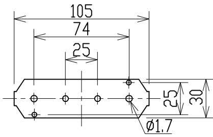
取付寸法(矢視 a) (縮尺1/3)
