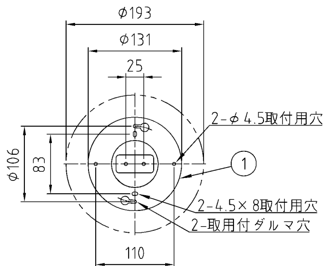
取付寸法（矢視a）
