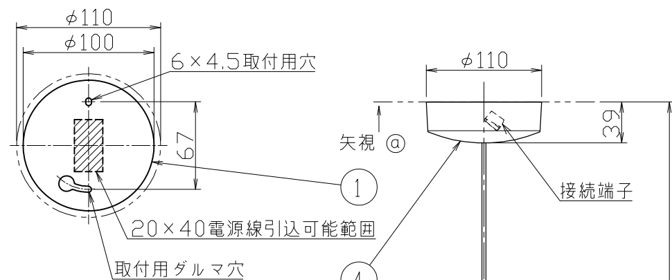
取付寸法（矢視 ①）
