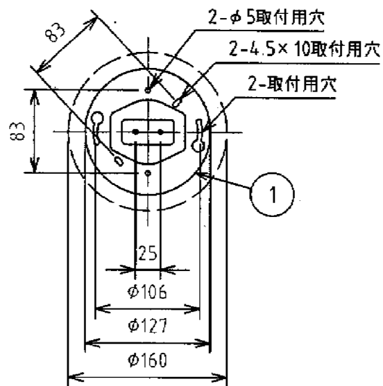
取付寸法 (矢視a)
