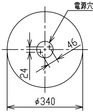
取付寸法(矢視①)
