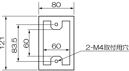
コンセントボックス取付面寸法図 (単位：mm)
