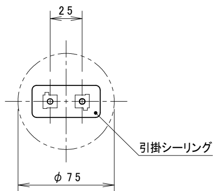
取付寸法(矢視a)
