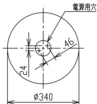
取付寸法(矢視 ㊦)
