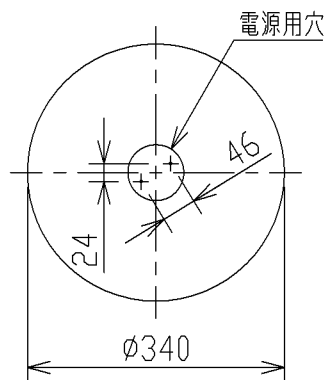
取付寸法(矢視 ㊸)
