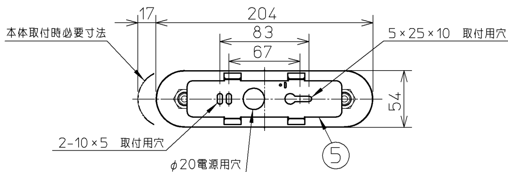
取付寸法 (矢視a)
