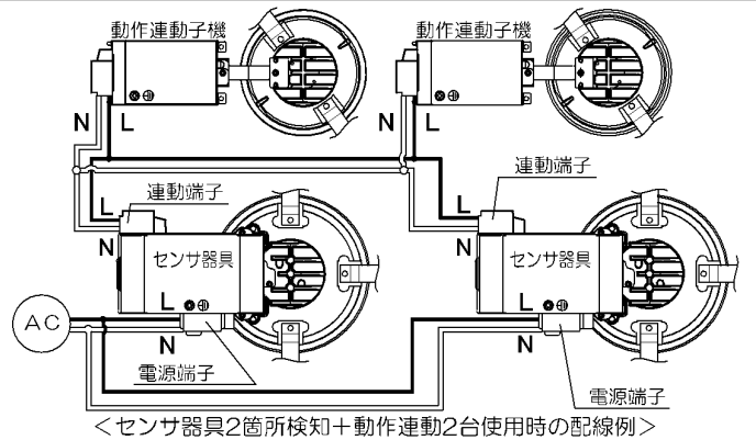
＜センサ器具2箇所検知＋動作連動2台使用時の配線例＞
