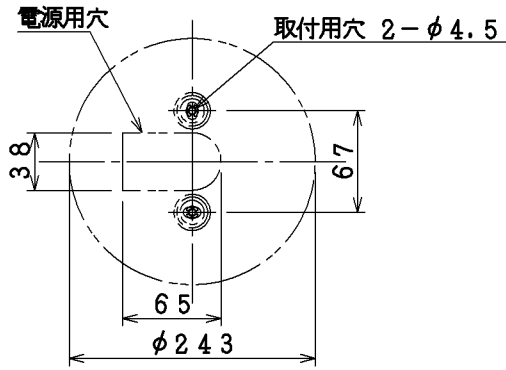
取付寸法(矢視⑧)
