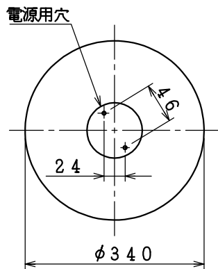
取付寸法(矢視④)
