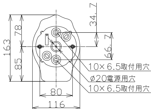
取付寸法 (矢視 ㊶)
