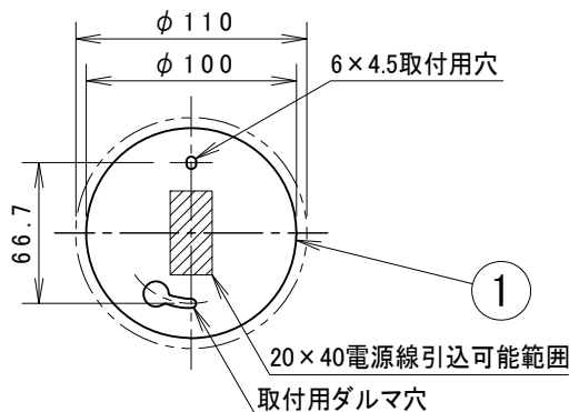
取付寸法(矢視a) (縮尺1/4)
