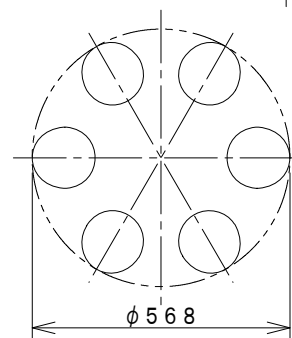
灯具配置図
