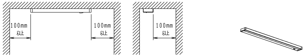
取付寸法 壁付の場合(矢視 ㉓)
