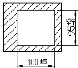
壁の穴あけ寸法
