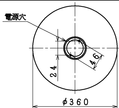
取付寸法 (矢視 ②)
