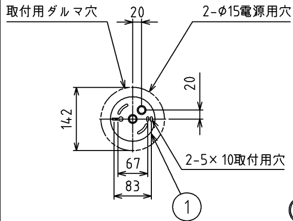
取付寸法 (矢視 a)
