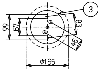
取付寸法 (矢視 α)
