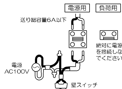
【送り配線(動作連動をさせない場合)】
