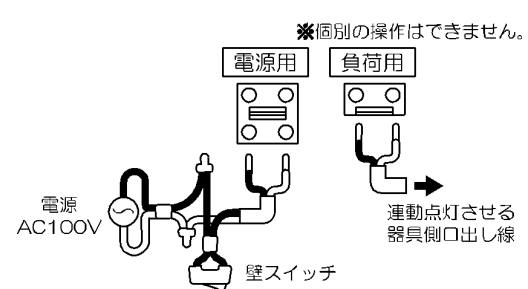
【送り配線(動作連動をさせる場合)】
