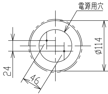
取付寸法(矢視 ②)
