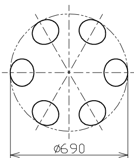
灯具配置図
