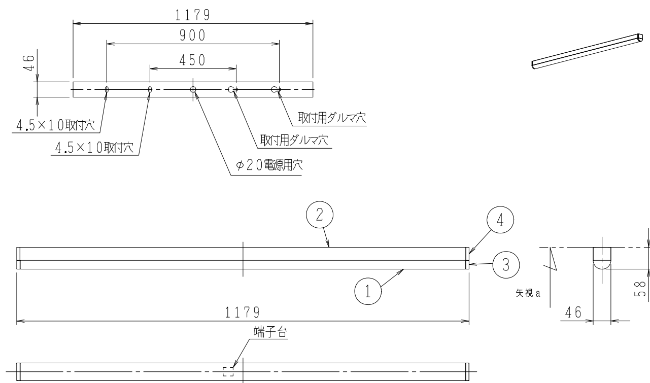
取付寸法（矢視 ④）
