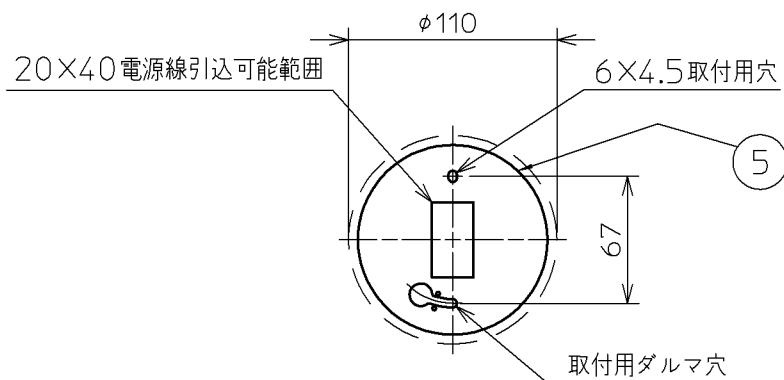
取付寸法(矢視 ㊤)
