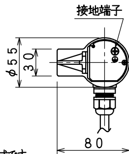
取付寸法(矢视图②)
