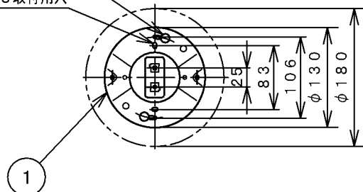
取付寸法 (矢視 a)
