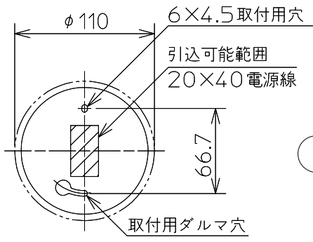
取付寸法 矢視a
