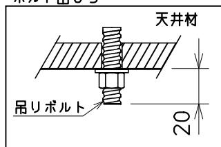
ボルト出し
