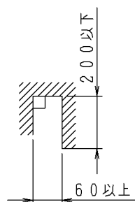
灯具最小施工寸法
