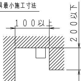
灯具最小施工寸法
