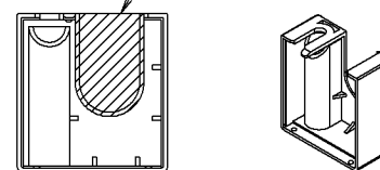
ノックアウト穴
