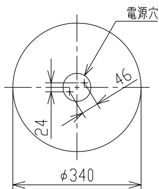
取付寸法(矢視 ②)
