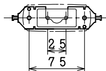
取付寸法(矢視④) S=1/5
