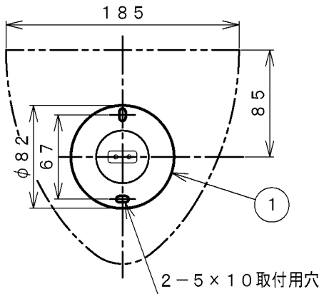
取付寸法 (矢視 a)
