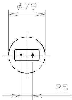
取付寸法 (矢視 ㉑)
