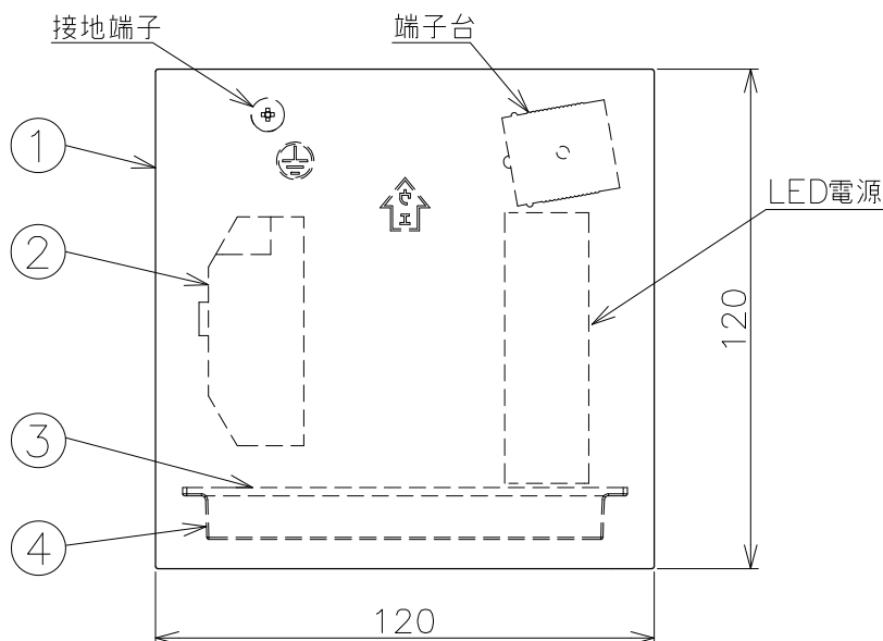
取付寸法
