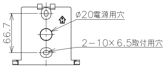
取付寸法
