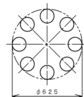
灯具配置図
