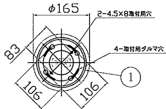
取付寸法(矢視 ①)
