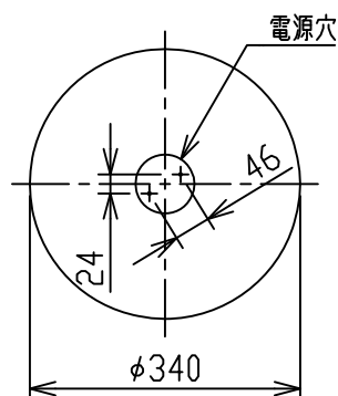
取付寸法(矢視 ㊶)
