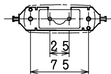
取付寸法(矢視⑨) S=1/5
