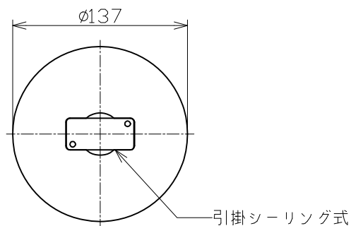
取付寸法 (矢視 (a))
