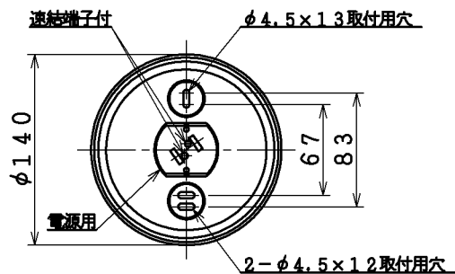
取付寸法(矢視 ⑧)
