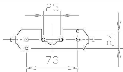
取付寸法 (矢視 ㊦)
