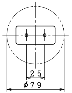
取付寸法(矢視 ㊸)
