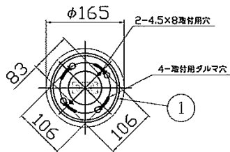
取付寸法(矢視 ①)
