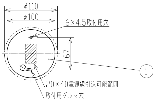
取付寸法(矢視a) (縮尺1/4)
