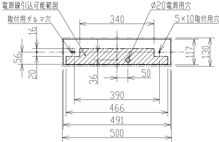
取付寸法(矢視a) (縮尺1/10)
